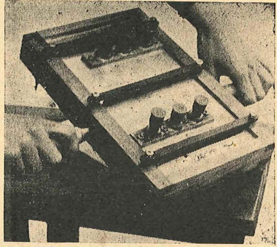
A gauche : le limographe 21 × 27
